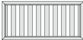
Zaunfeld 1.800 x 850 mm 10 Latten
